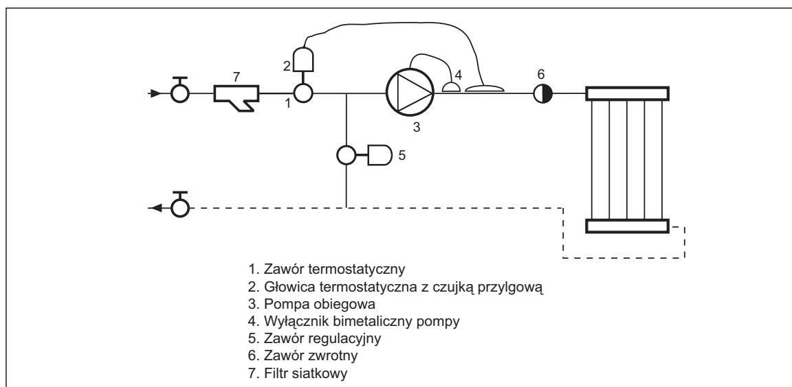
Rys. 70. Przykład rozwiązania węzła mieszającego
