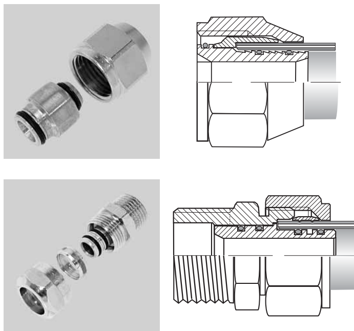
Rys. 15. Przekroje złączek VESTOL i VESTOL ZBK
