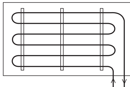
Rys. 47. Wężownica w układzie poziomym meandrowym w ogrzewaniu ściennym
