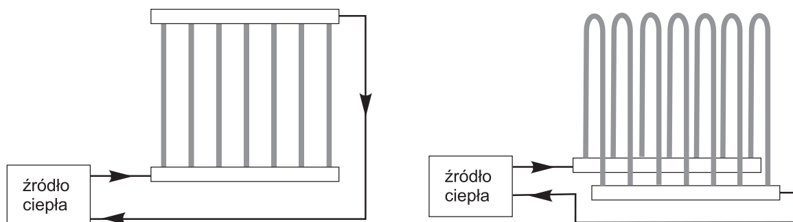
Rys. 73 i rys. 74. Przykłady rozwiązań układów Tichelmana
