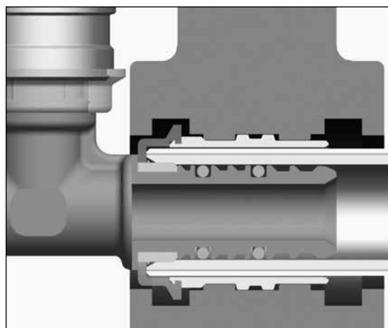
Rys. 9. Pozycjonowanie szczęki typu TH na złączce typu Kisan WL
