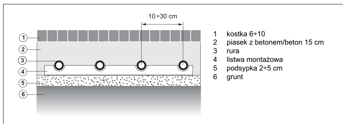
Rys. 71. Ogrzewanie powierzchni z kostką
