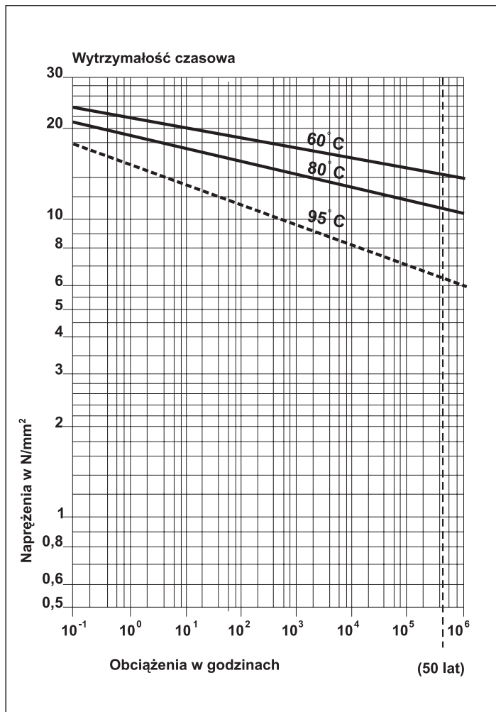
Rys. 2. Wykres wytrzymałości czasowej rur wielowarstwowych
