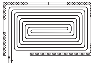
Rys. 38. Wężownica ułożona w kształcie ślimaka
