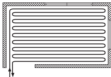
Rys. 37. Wężownica ułożona w kształcie meandru
