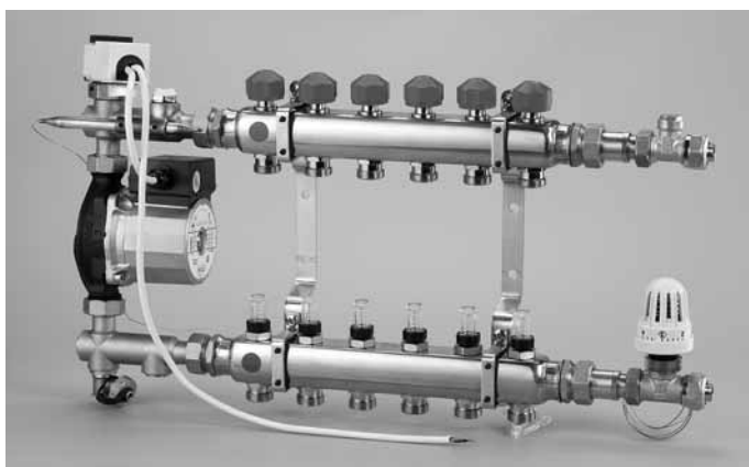
Rys. 61. Układ mieszający UMR KISAN COMFORT
