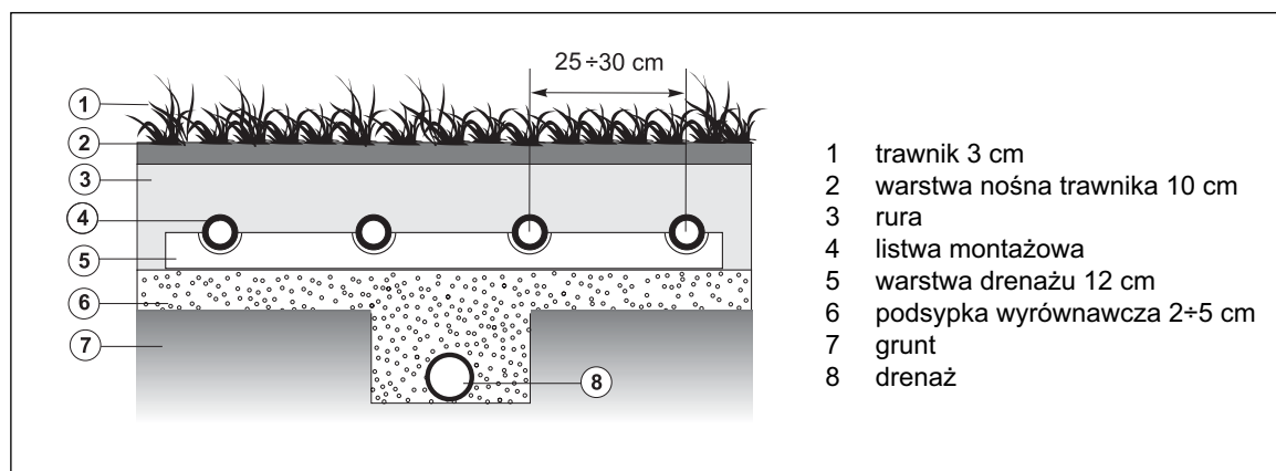
Rys. 72. Ogrzewanie boiska
