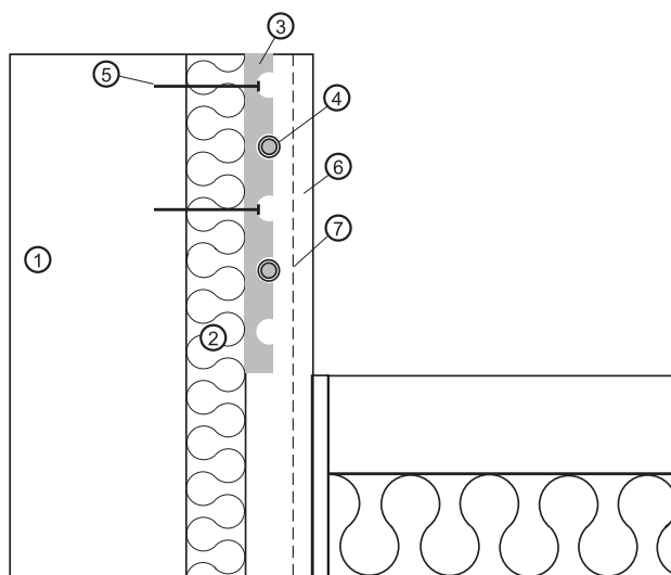
Rys. 49. Przekrój połączenie ogrzewania ściennego z ogrzewaniem podłogowym
