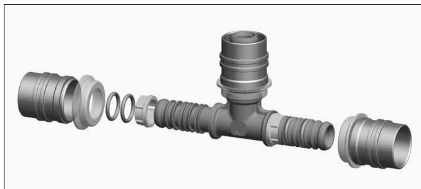
Rys. 3. Złączka zaprasowywana typu Kisan WL
