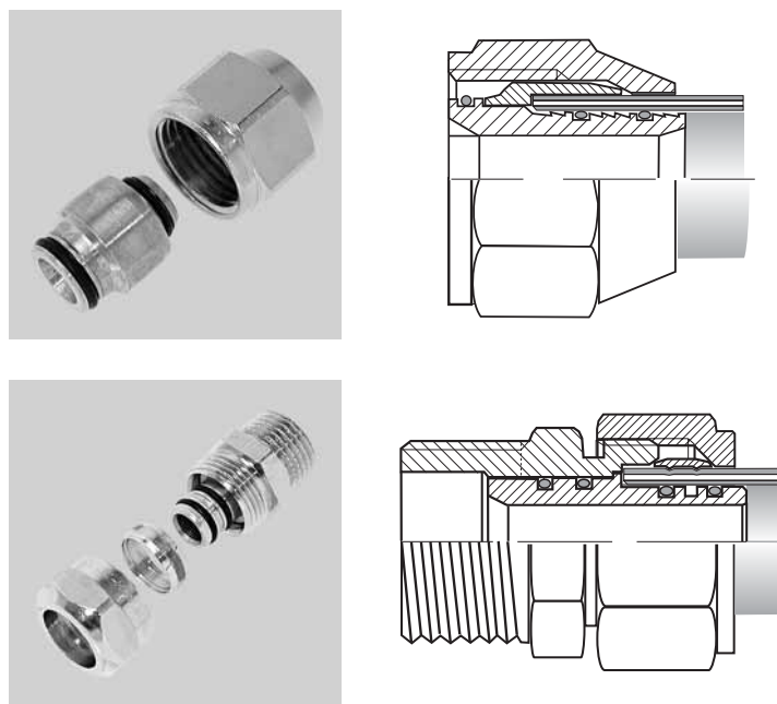
Rys. 6. Złączki zaciskowe typu Vestol i Vestol ZBK
