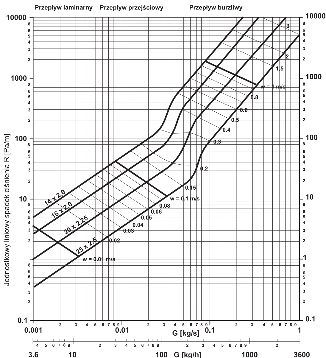
Rys. 24. Jednostkowy liniowy spadek ciśnienia R dla instalacji wodociągowych
