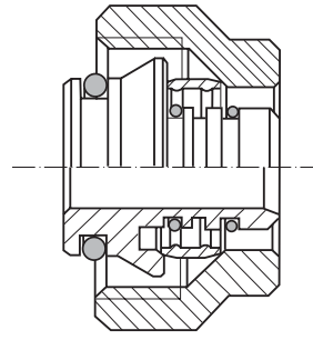
Rys. 7. Złączka przygrzejnikowa typu G \frac{3}{4} " Eurokonus
