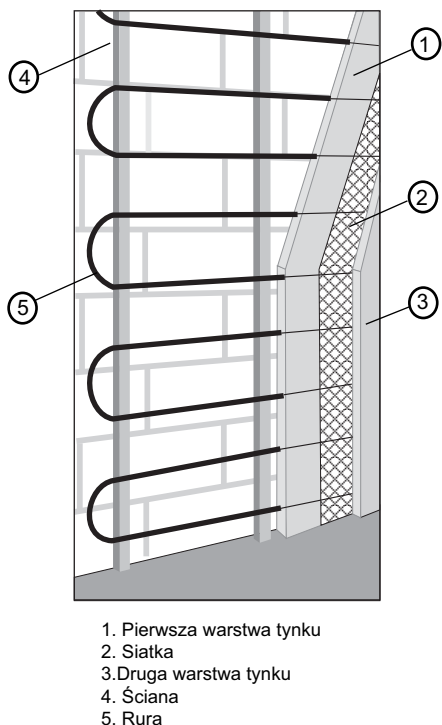
Rys. 46. Przekrój ogrzewania ściennego z tynkiem nakładanym dwuwarstwowo
