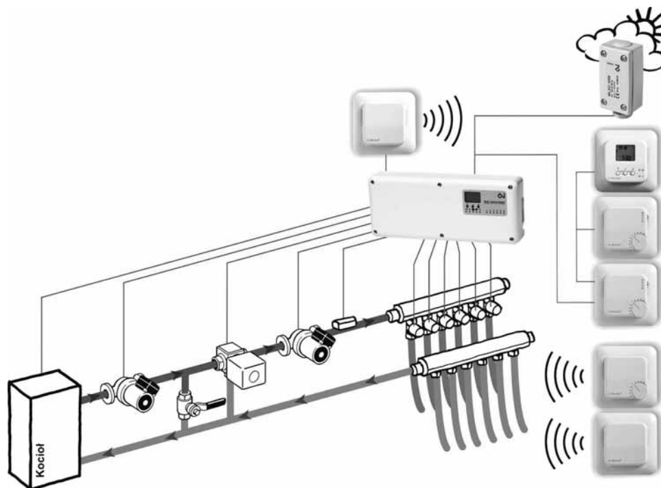
Rys. 67. Schemat podłączenia systemu cyfrowego WLM II – KISAN COMFORT DIGITAL CONTROL
