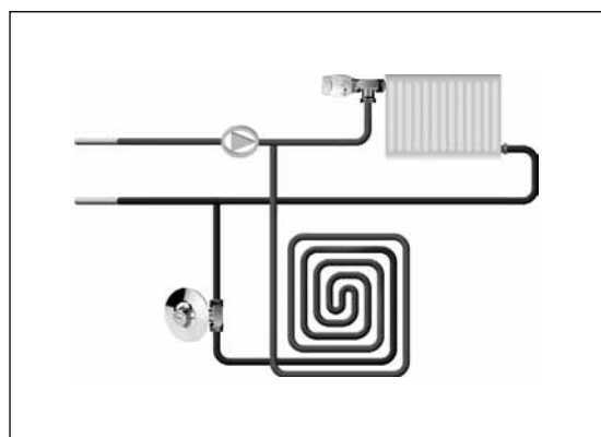
Rys. 63. Zawór typu RTL w formie modułu ściennego
