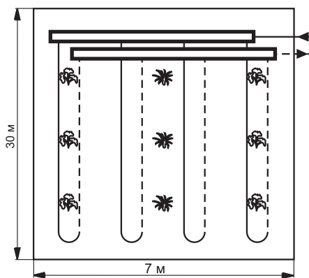
Rys. 68. Układ pętli
