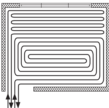
Rys. 39. Wężownice ułożone ze strefą brzegową na oddzielnej pętli
