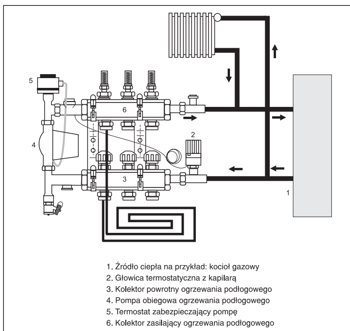
Rys. 60. Schemat układu mieszającego dołączanego do rozdzielacza
