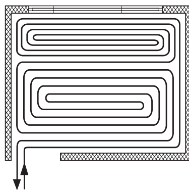
Rys. 40. Wężownice ułożone ze strefą brzegową na jednej pętli
