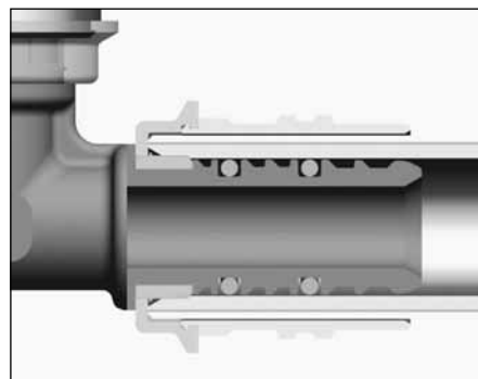
Rys. 4. Przekrój złącza zaprasowywanego typu Kisan WL
