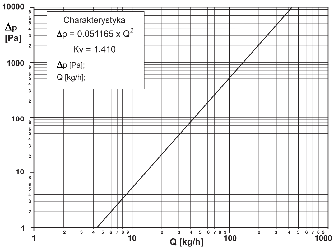
Rys. 57. Charakterystyka rozdzielacza zasilającego z zaworami odcinającymi
