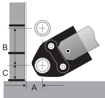
Rys. 14. Odległości od ścian, podłóg i sąsiednich rurociągów
