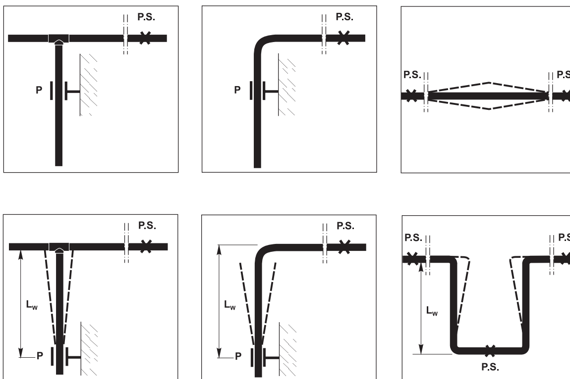
Rys. 21. Przykłady rozwiązań kompensacji rurociągów
