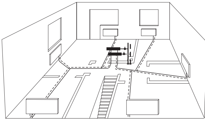
Rys. 29. Rozprowadzenie przewodów z trójnikami w przegrodach poziomych – dopuszczalne przy stosowaniu złączek zaprasowywanych
