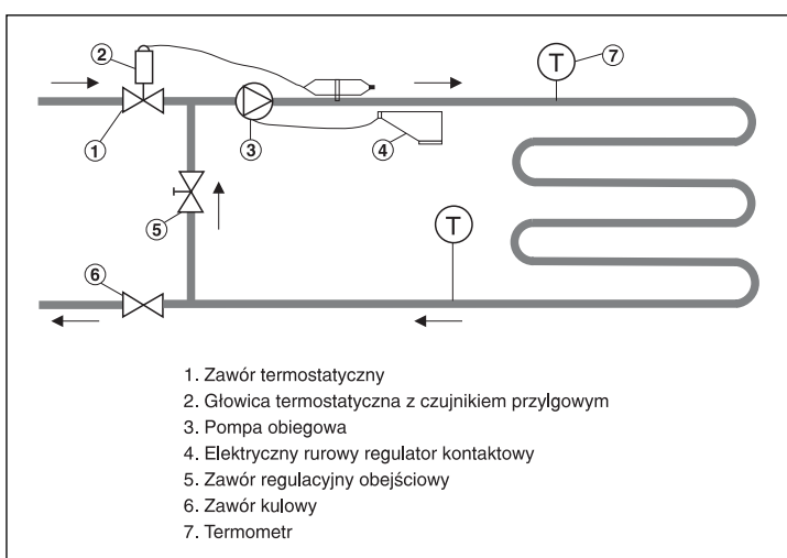
Rys. 59. Schemat układu mieszającego do samodzielnego montażu
