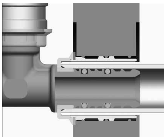
Rys. 8. Pozycjonowanie szczęki typu KI na złączce typu Kisan WL.
