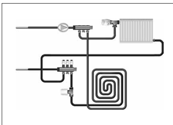
Rys. 62. Zawór typu RTL zamontowany przy rozdzielaczu
