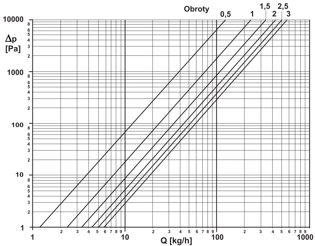
Rys. 56. Charakterystyka rozdzielacza powrotnego z zaworami do regulacji wstępnej
