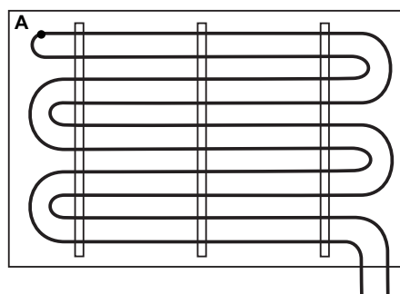
Rys. 48. Wężownica w układzie podwójnego meandru
