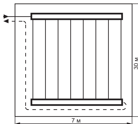
Rys. 69. Układ współprądowy
