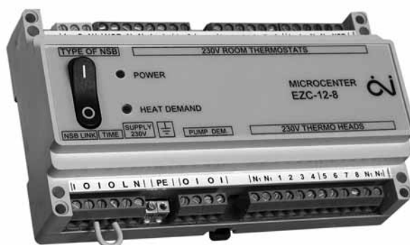
Rys. 65. Listwa sterująca EZC z przekaźnikami pompy i kotła
