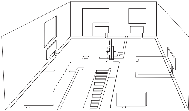
Rys. 28. Rozprowadzenie przewodów w pętli jednorurowej
