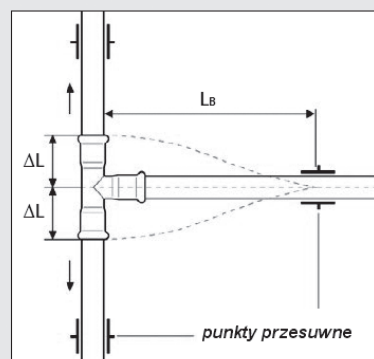
Rys. 14 Kompensator T-kształtowy
