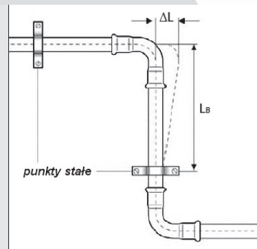
Rys. 13 Kompensator wydłużeń Z-kształtowy
