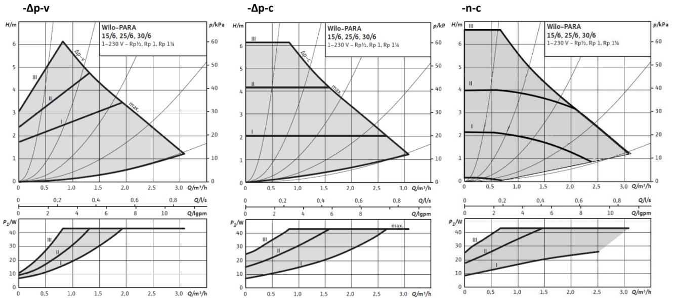
Charakterystyka pompy Wilo PARA RS 15/6
