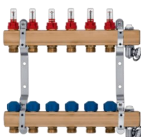
KRPT – Rozdzielacz 1" do ogrzewań płaszczyznowych i grzejnikowych z wyjściem do złączek G 3/4" o standardzie Eurokonus
