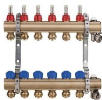
KRPT – Rozdzielacz 1" do ogrzewań płaszczyznowych i grzejnikowych ze złączkami Eurokonus G 3/4" x 16 x 2
