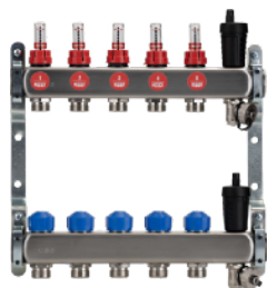
KRIPT – Rozdzielacz 1" ze stali nierdzewnej
